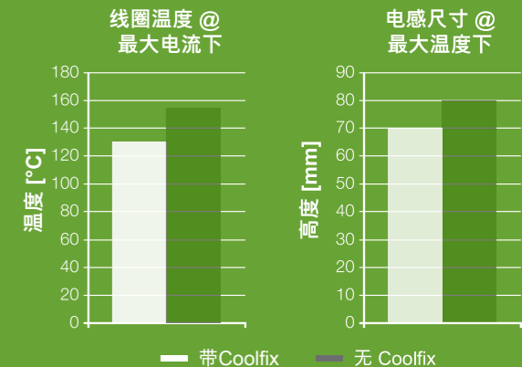
测试分析使用 Ø120 mm, ~5 kg 罐形电感器。
