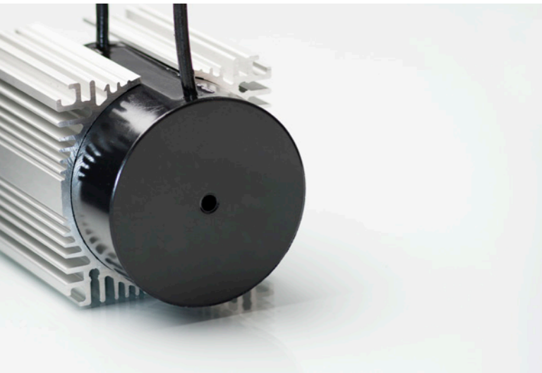
Coolfix 充分利用罐装电感的外形结构，增加了安装和冷却效率。
