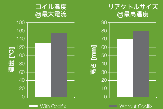
Ø120 mm, 5 kg Inductitにてテスト。
